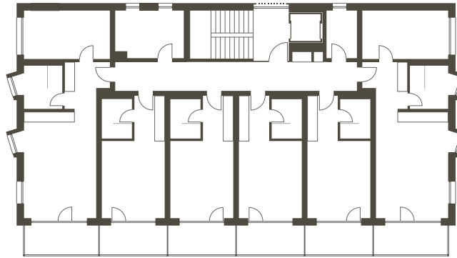
Grundriss 1./2. Obergeschoss
